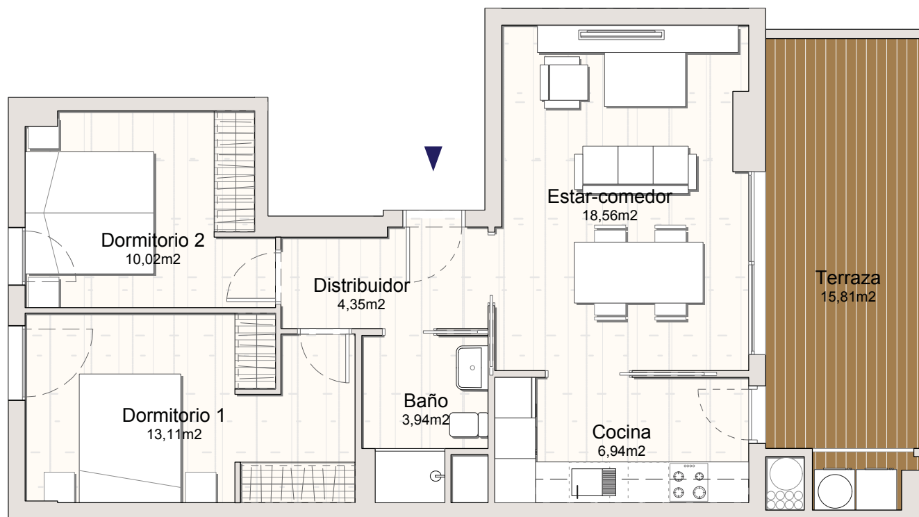
PLANTA 2 _ PUERTA 2
