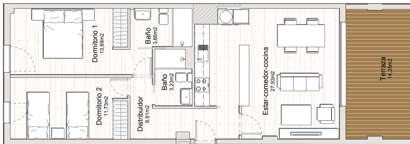
PLANTA 5 _ PUERTA 4
